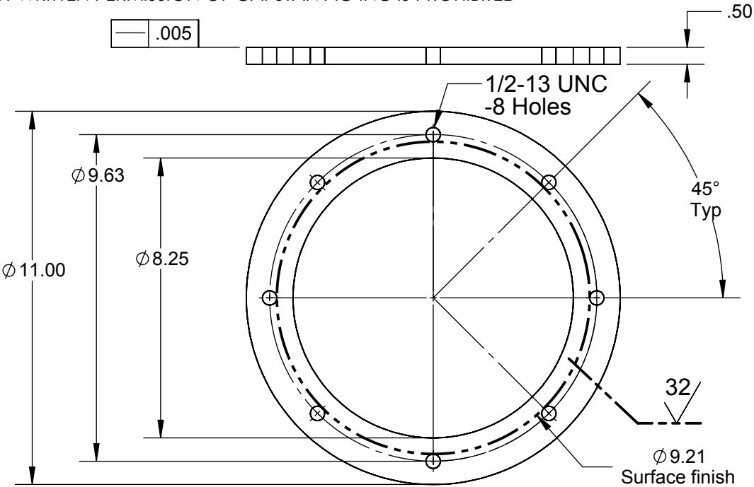
Top Flange A36 Steel
