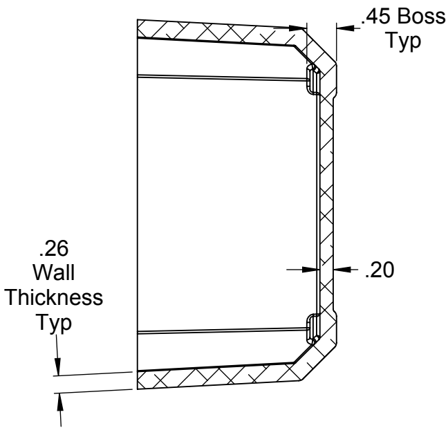
SECTION G-G SCALE 1 : 2
