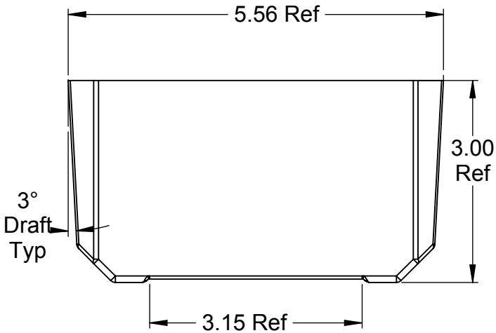
SECTION G-G SCALE 1 : 2
